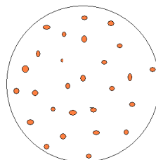
7. The «Big Bang»
